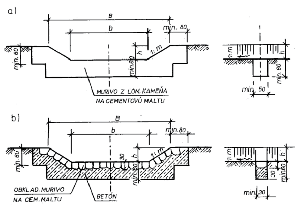
Pásky a) kamenný, b) betónový
