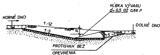
Sklz s vývarom (podľa Kališa)
